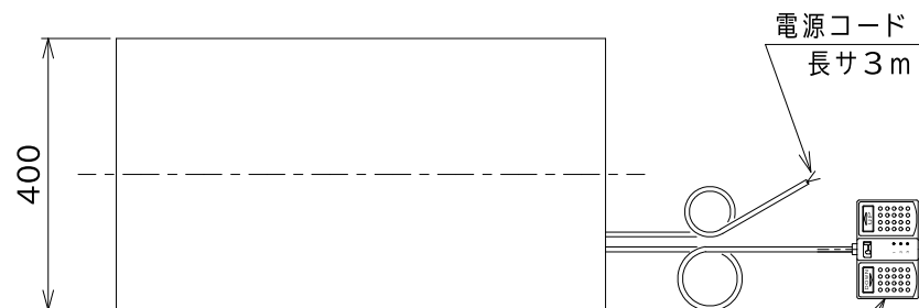
フットスイッチ (UP・DOWN) コード長さ2m
